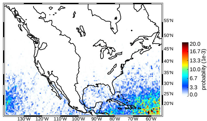
(d) MAM broad stratiform regions strong thresholds
