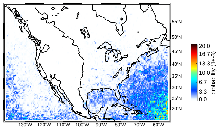
(d) JJA broad stratiform regions moderate thresholds
