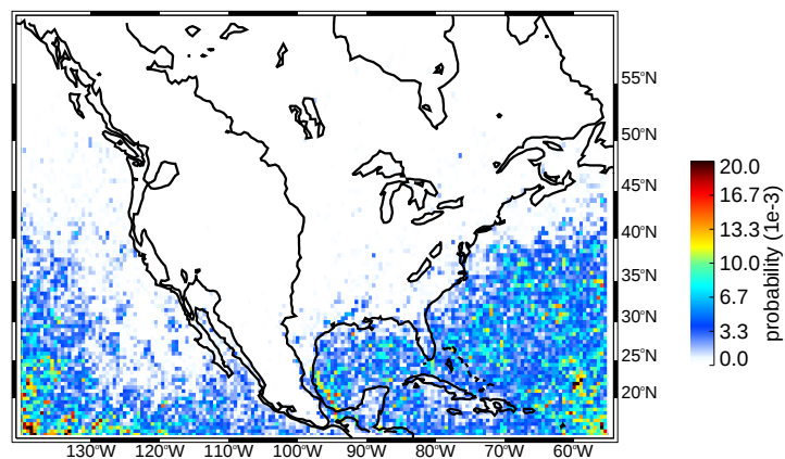
(d) SON broad stratiform regions moderate thresholds
