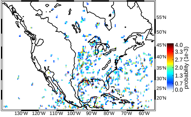
(d) SON wide convective cores
