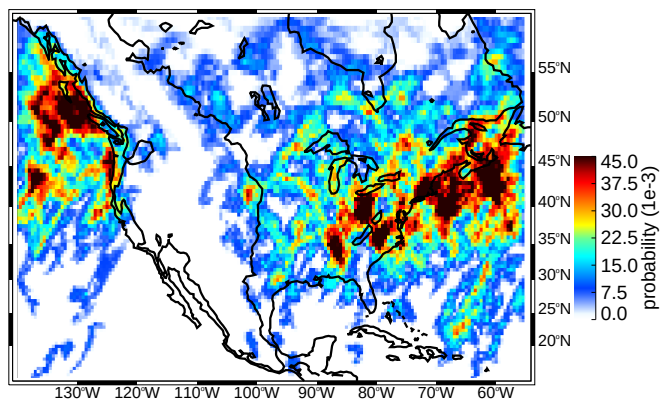
(a) MAM broad stratiform regions
