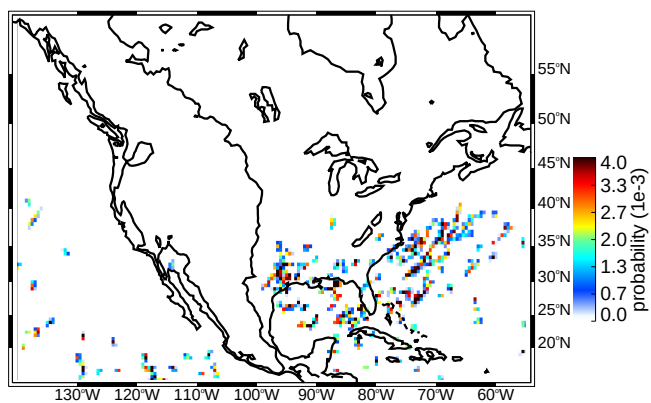
(d) DJF wide convective cores
