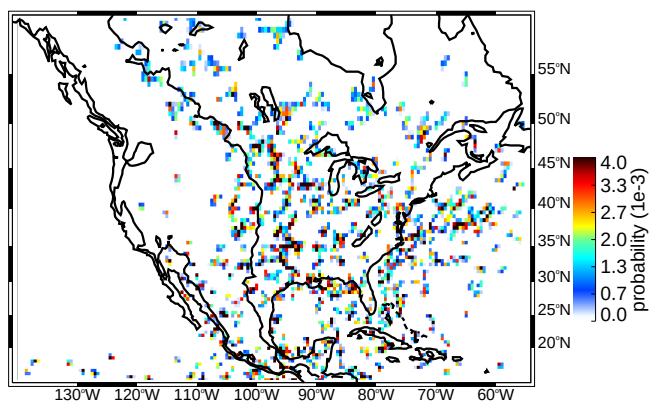
(d) JJA wide convective cores
