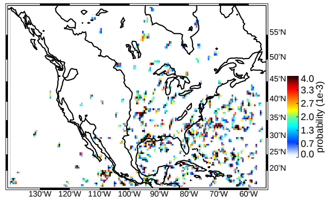
(d) SON wide convective cores strong thresholds (uw)
