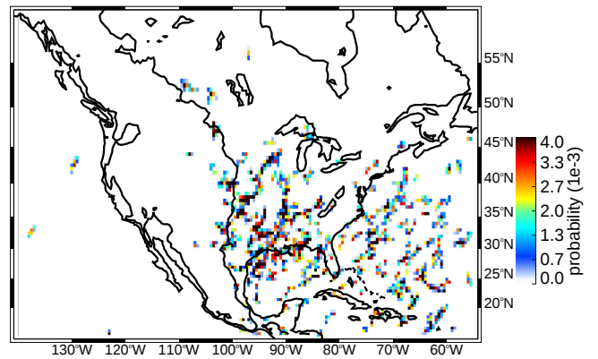
(d) MAM wide convective cores strong thresholds (uw)
