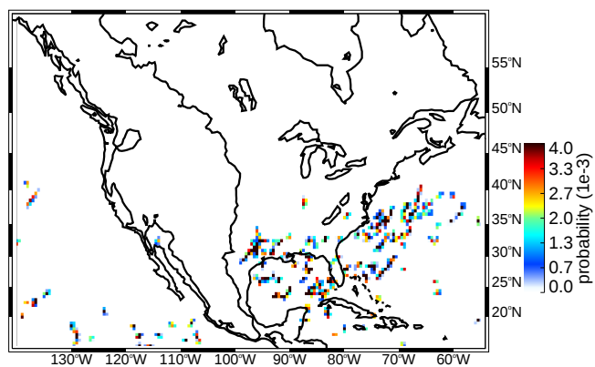
(d) DJF wide convective cores strong thresholds (uw)
