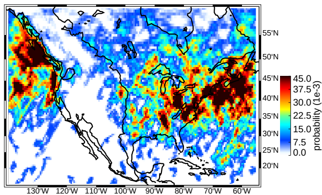
(a) MAM broad stratiform regions
