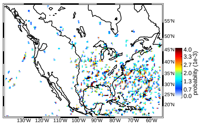
(d) MAM wide convective cores
