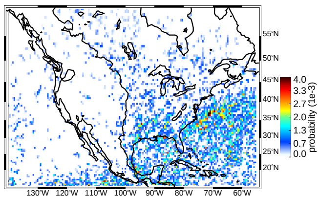
(d) J-D wide convective cores
