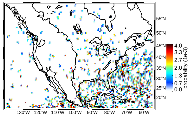
(d) SON wide convective cores moderate thresholds (uw)
