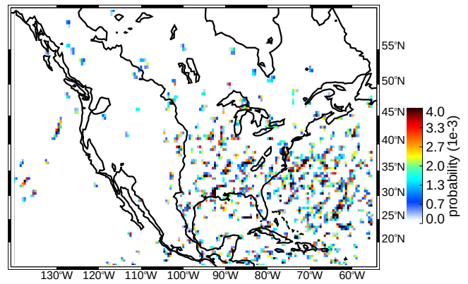
(d) MAM wide convective cores moderate thresholds (uw)
