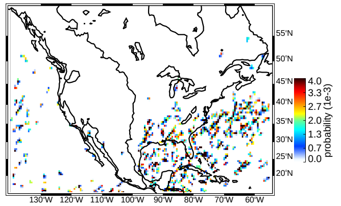
(d) DJF wide convective cores moderate thresholds (uw)
