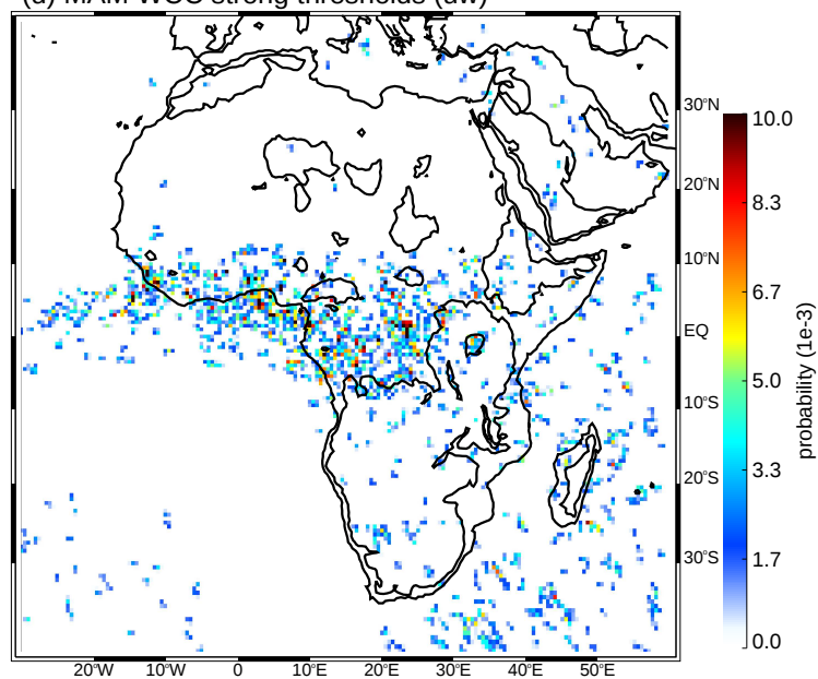
(d) MAM WCC strong thresholds (uw)
