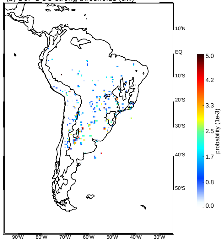
(d) DJF WCC strong thresholds (uw)
