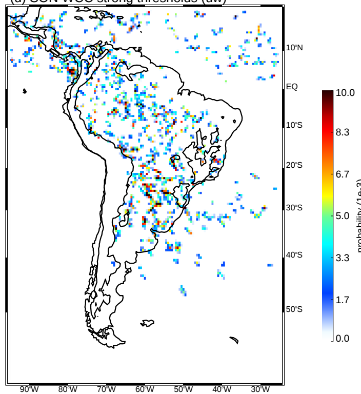
(d) SON WCC strong thresholds (uw)
