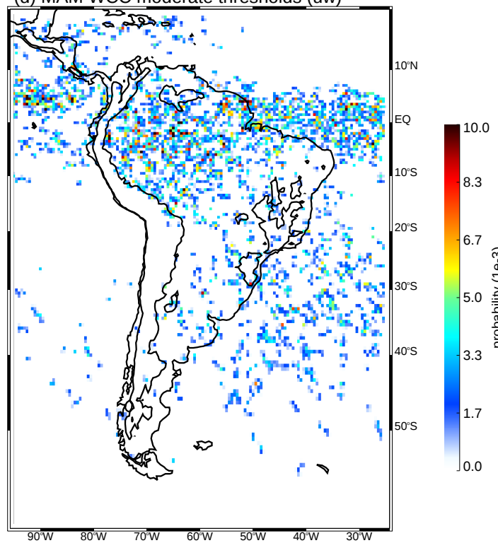
(d) MAM WCC moderate thresholds (uw)
