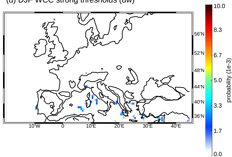
(d) DJF WCC strong thresholds (uw)
