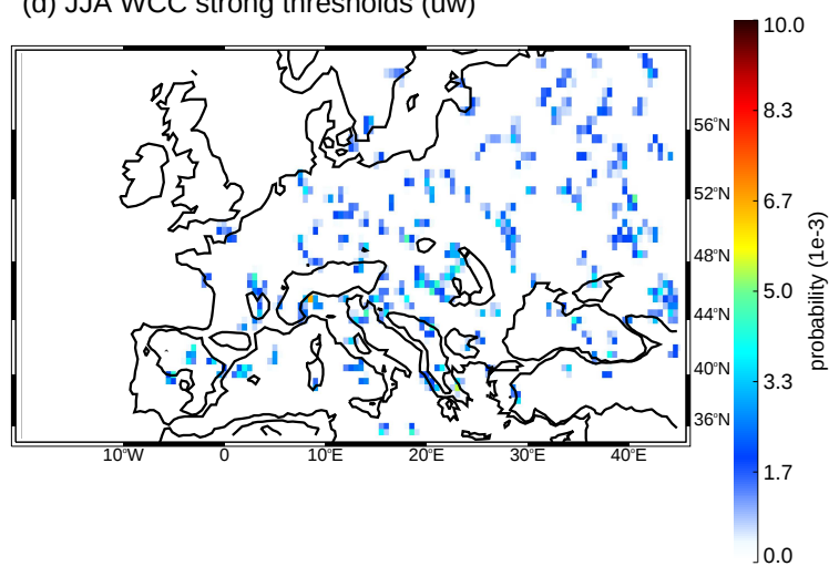
(d) JJA WCC strong thresholds (uw)
