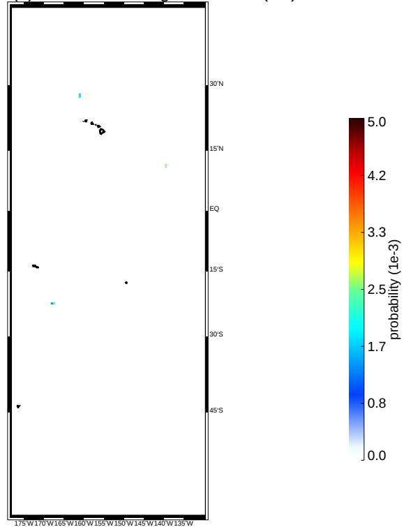
(d) DJF WCC strong thresholds (uw)
