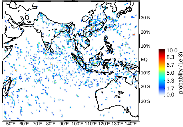
(d) MAM WCC strong thresholds (uw)
