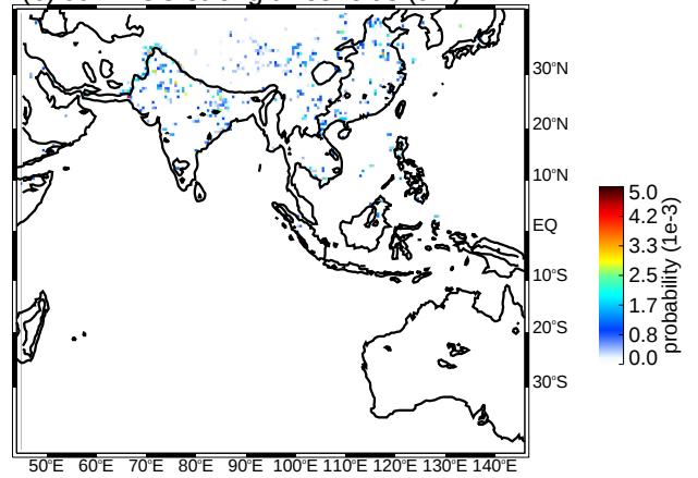
(d) JJA WCC strong thresholds (uw)
