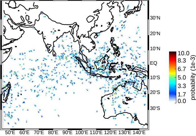
(d) DJF WCC strong thresholds (uw)
