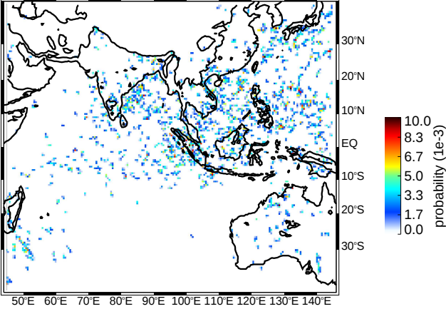
(d) SON WCC strong thresholds (uw)
