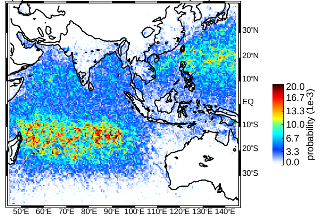
(d) SON broad stratiform regions strong thresholds (uw)
