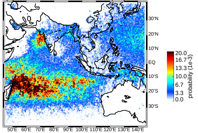
(d) JJA broad stratiform regions strong thresholds (uw)
