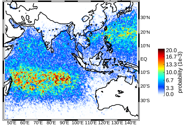
(d) SON broad stratiform regions moderate thresholds (uw)
