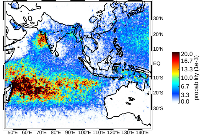
(d) JJA broad stratiform regions moderate thresholds (uw)
