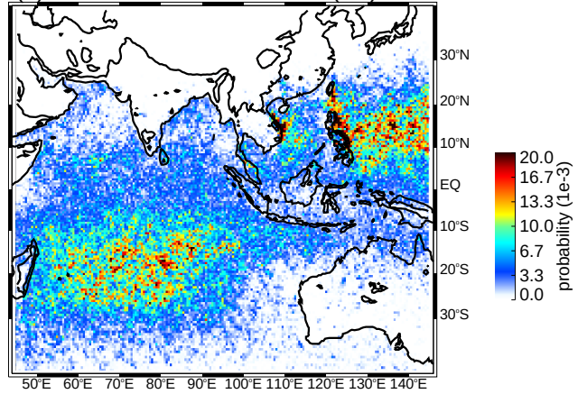
(d) DJF broad stratiform regions moderate thresholds (uw)
