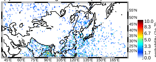
(d) JJA WCC strong thresholds (uw)
