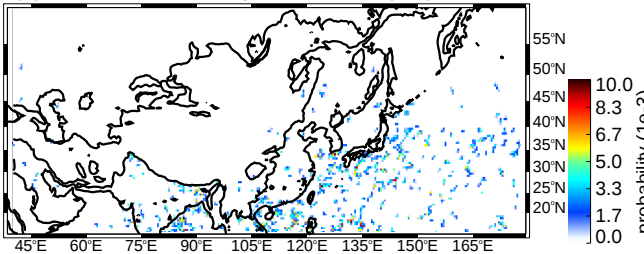
(d) SON WCC strong thresholds (uw)
