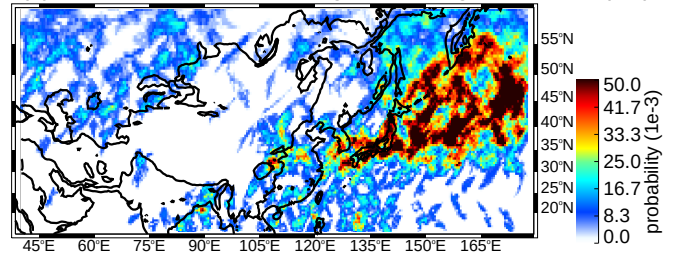
(d) SON broad stratiform regions strong thresholds (uw)
