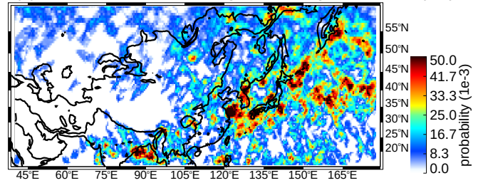
(d) JJA broad stratiform regions strong thresholds (uw)
