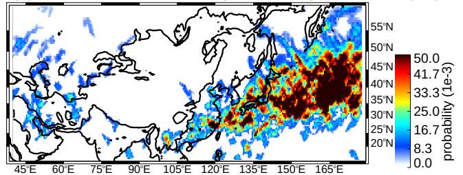
(d) DJF broad stratiform regions strong thresholds (uw)
