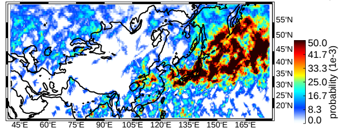
(d) SON broad stratiform regions moderate thresholds (uw)
