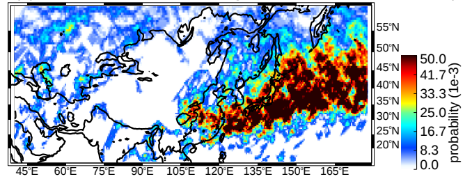
(d) MAM broad stratiform regions moderate thresholds (uw)
