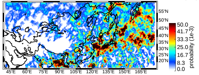
(d) JJA broad stratiform regions moderate thresholds (uw)
