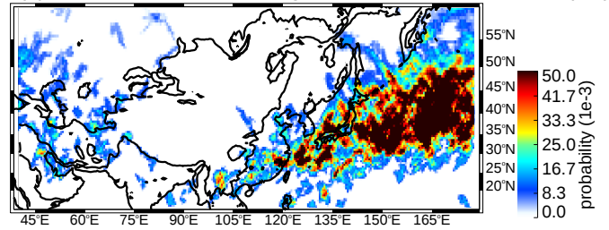
(d) DJF broad stratiform regions moderate thresholds (uw)
