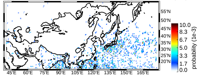
(d) SON wide convective cores strong thresholds (uw)
