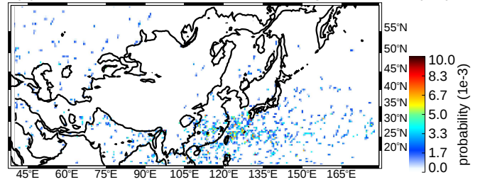
(d) MAM wide convective cores strong thresholds (uw)
