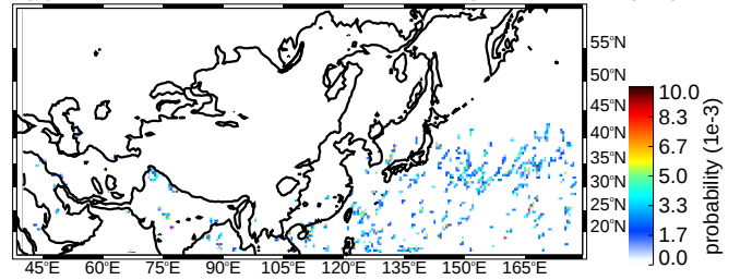
(d) DJF wide convective cores strong thresholds (uw)
