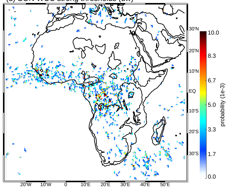
(d) SON WCC strong thresholds (uw)
