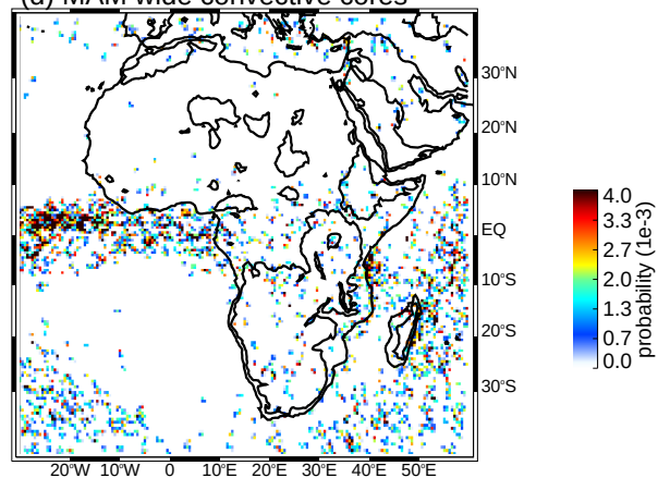
(d) MAM wide convective cores
